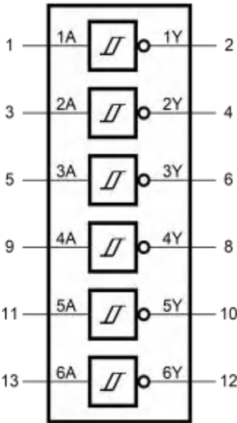
图 1 逻辑符号
