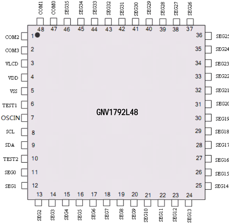
LQFP48
