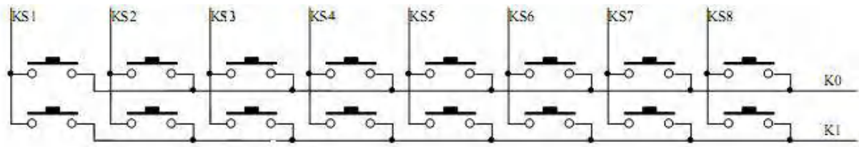
图 4、键扫矩阵
